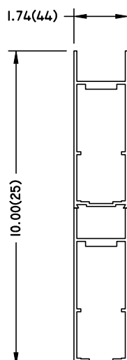
10" MUNTIN BAR
