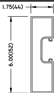
JAMB-6"
