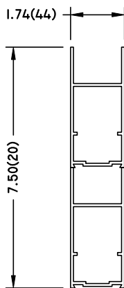
8" NOMINAL MUNTIN BAR
